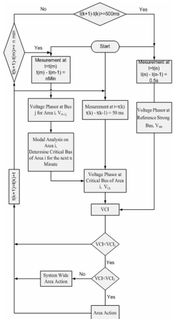
شکل ۱۷- فلوچارت الگوریتم VCI
